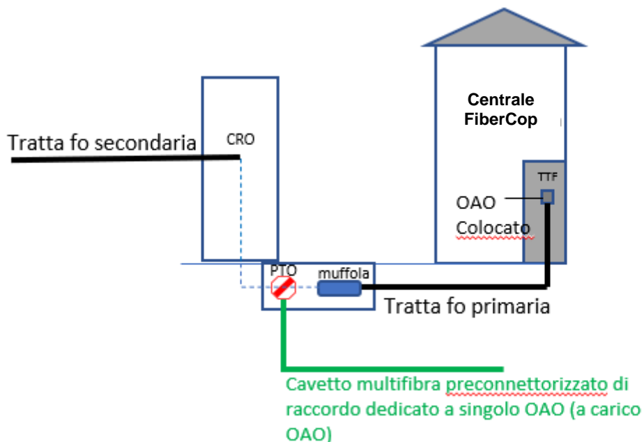
Figura 5: Esempio di PTO senza minipozzetto in architettura CRO
