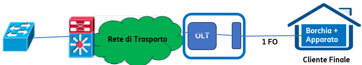
Figura 1: Schema impiantistico FTTO per velocità inferiori o uguali a 1 Gbps
