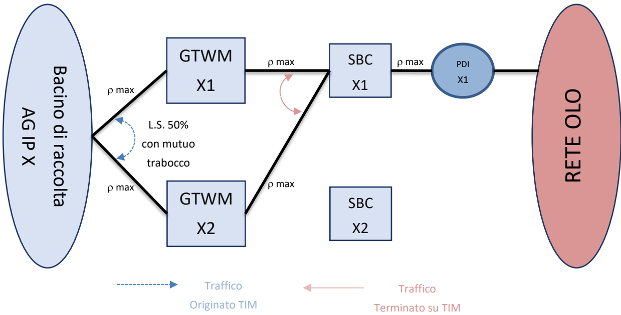
Figura 4: Criteri di dimensionamento dei moduli CAC: attestazione a Pdi singolo
