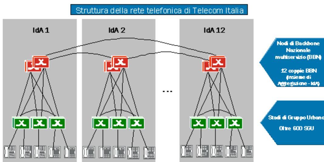
Figura 1: Architettura dell'interconnessione TDM/ISUP
