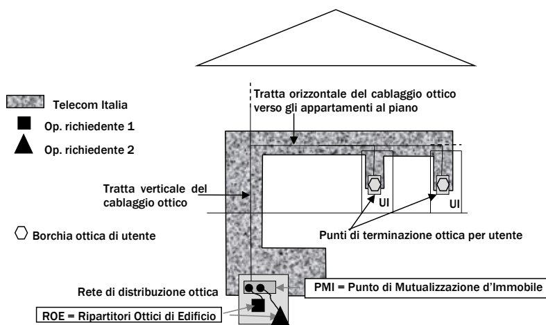
Figura 3: Architettura per la fornitura del servizio Segmento di Terminazione in Fibra Ottica
