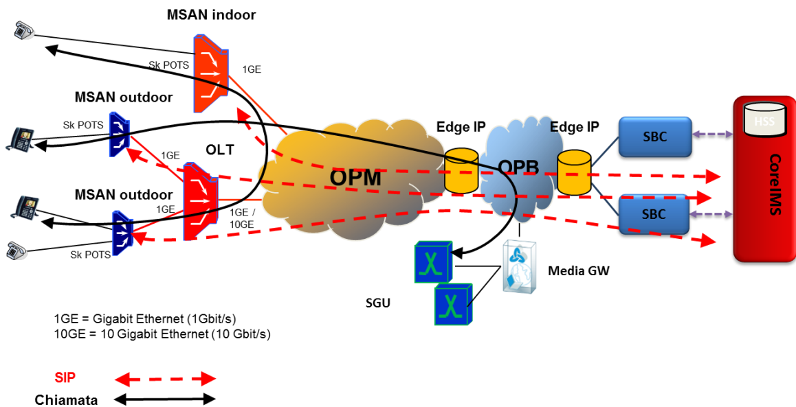
Figura 2 Architettura di rete MSAN H.248
