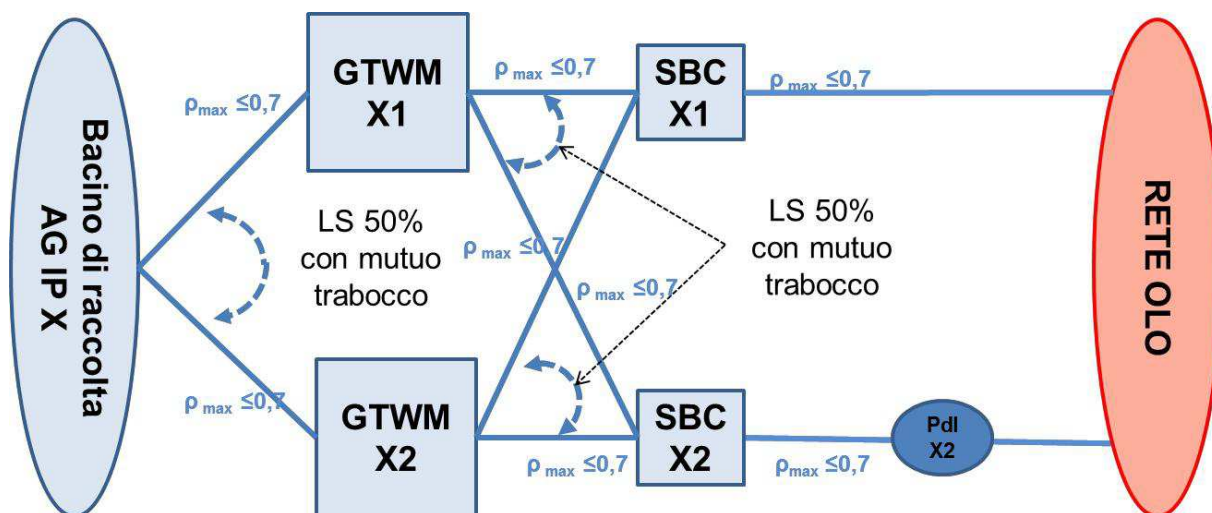
Figura 4: Criteri di dimensionamento delle risorse della rete IP
