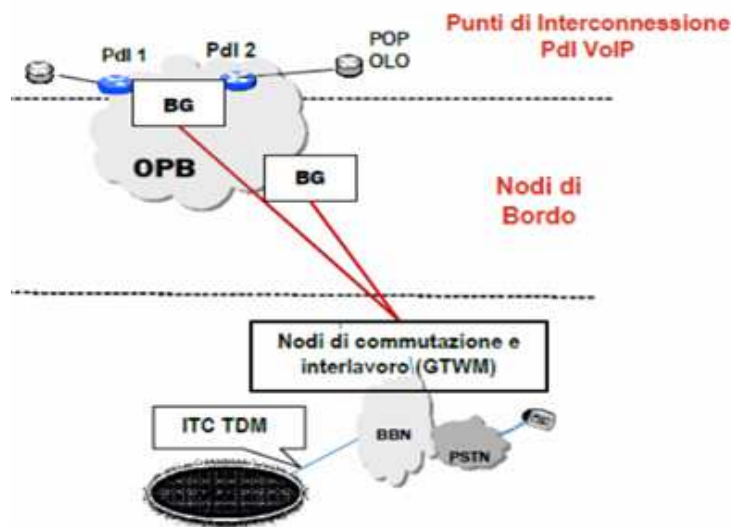
Figura 2: Architettura dell'interconnessione VoIP/IP
