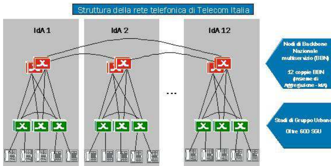
Figura 1: Architettura dell'interconnessione ISUP/TDM.
