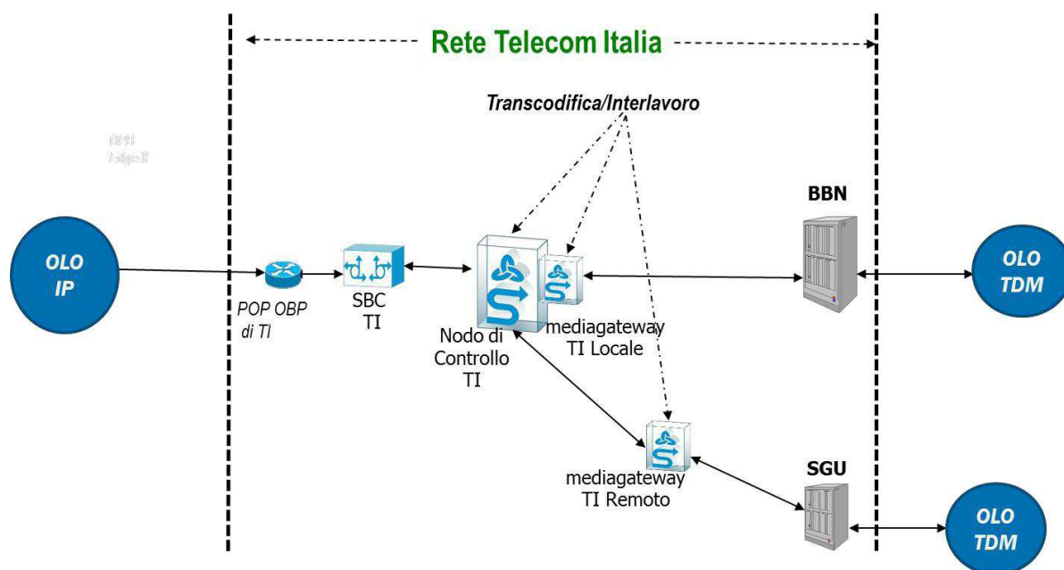
Figura 6: Catena impiantistica servizio di transito distrettuale misto
