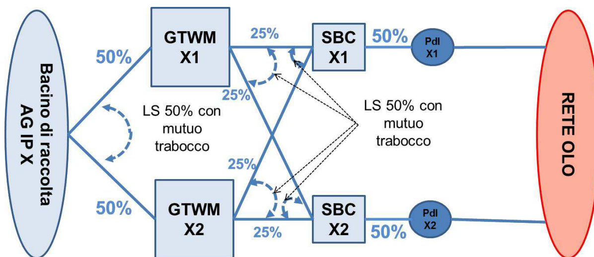
Figura 5: Criteri di Instradamento del traffico
