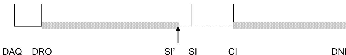
Figura 2: Tempi per il provisioning del servizio end-to-end validi ai fini dello SLA
