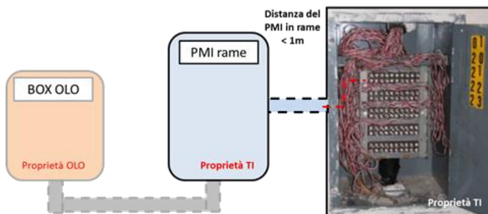
Figura 4: Schema operativo di massima per l'infrastruttura atta alla fornitura del Segmento di Terminazione in Rame
