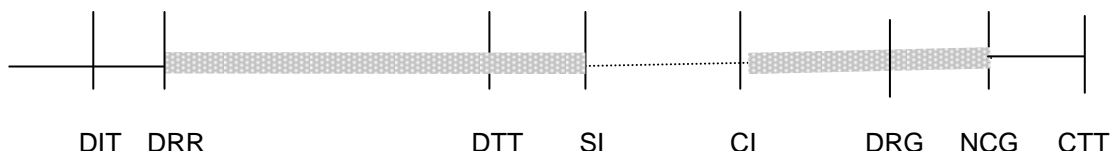
Figura 6: Tempi per il ripristino del servizio end-to-end
