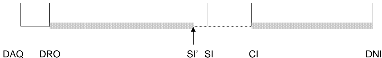
Figura 2: Tempi per il provisioning del servizio end-to-end validi ai fini dello SLA
