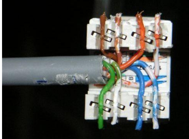
Figura 63 – Predisposizione dei conduttori su connettore femmina
