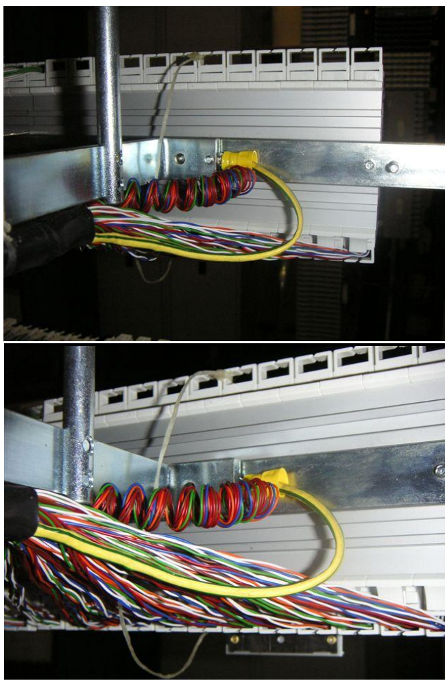
Figura 42 – Coppie di scorta avvolte in un'unica spiralina dietro la striscia IDC
