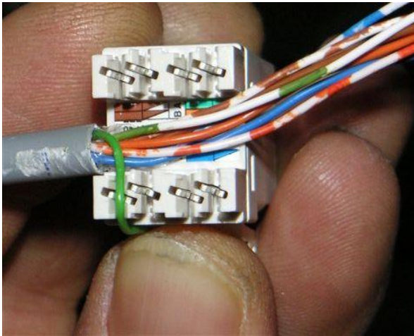
Figura 63 – Predisposizione dei conduttori su connettore femmina
