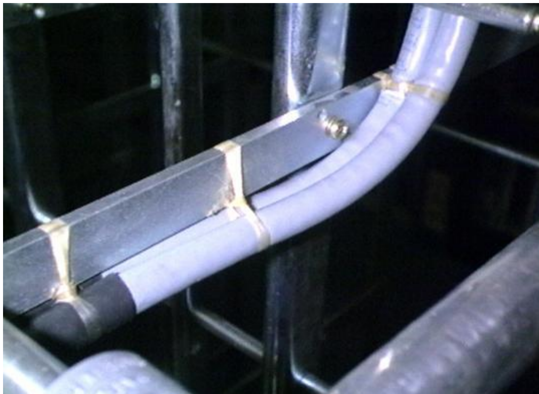
Figura 40 – Esempio di legatura dei cavi B.F. sul lato orizzontale del Ripartitore in prossimità della striscia di terminazione.
