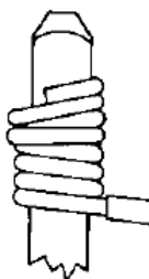
Figura 52 – Esempio di spire sovrapposte
