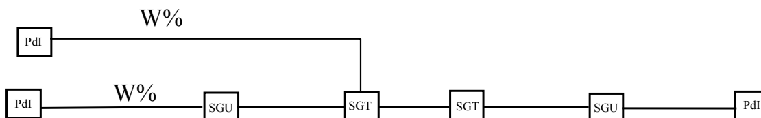
Figura 1 - Schema di riferimento di un collegamento Nazionale
